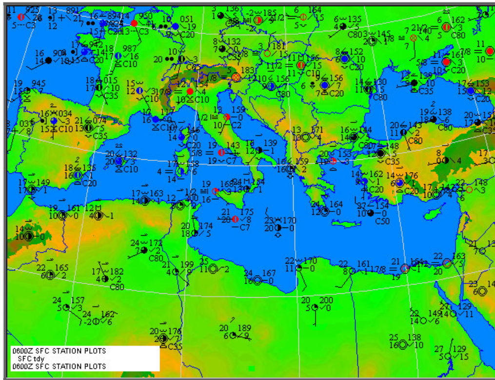
Σχήμα 1: Χάρτης με αναφορές μετεωρολογικών σταθμών.
